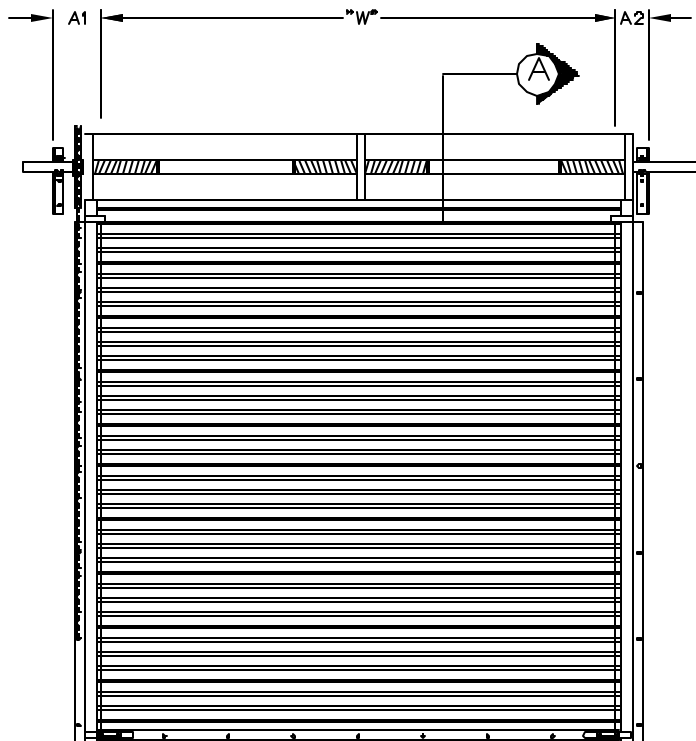
ELEVATION
