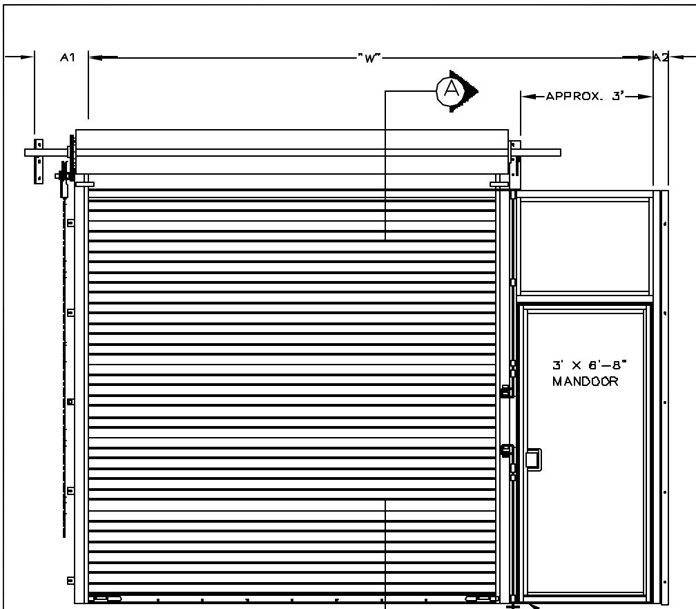
ELEVATION
